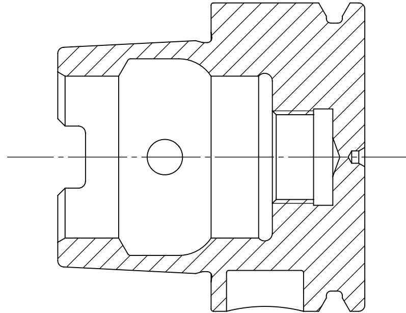
SCHNITT A-A (2 : 1)
