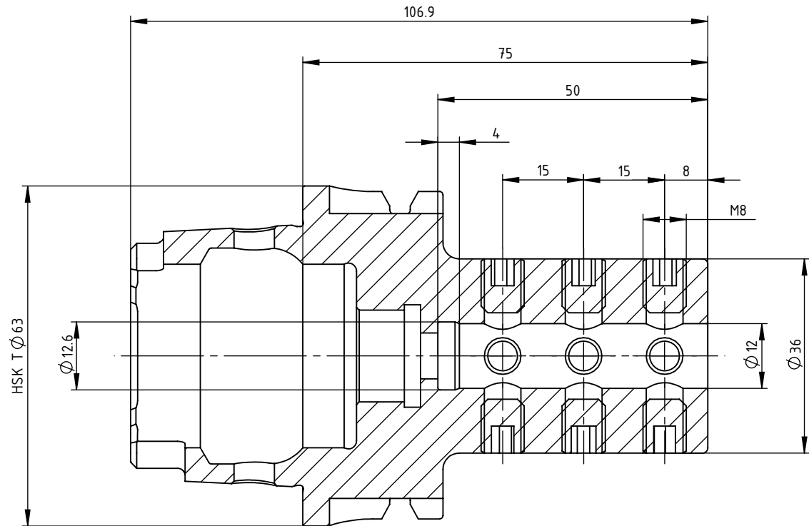
SCHNITT A-A
