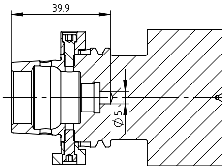
SCHNITT B-B (1 : 1.5)
