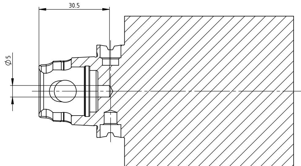
SCHNITT A-A (1 : 1)
