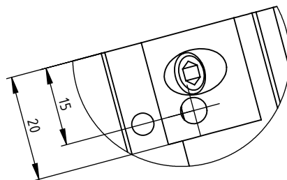
ANSICHT A (1 : 1)
