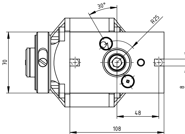
ANSICHT B
