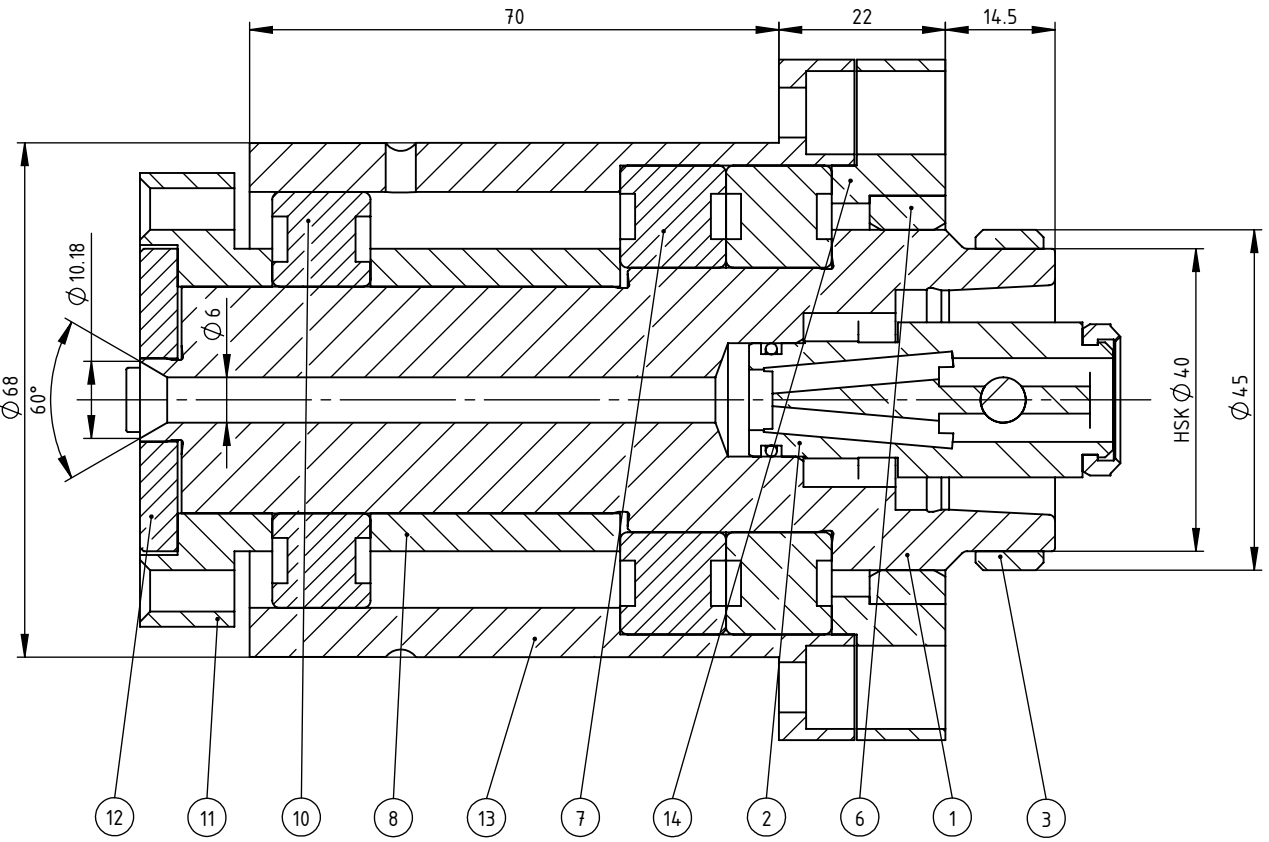
SCHNITT A-A (1 : 1)
